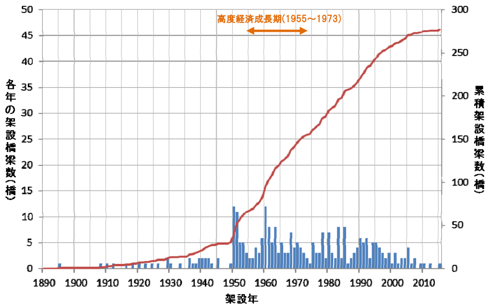
図13 橋梁架設年の分布
