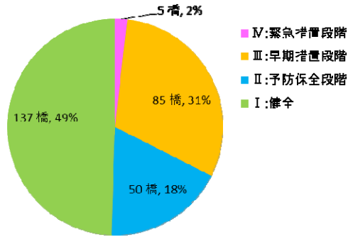
図 15 管理橋の健全性の状況 (平成 28 年 3 月現在)
