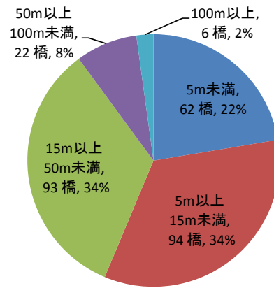
図8 橋長別橋梁数
