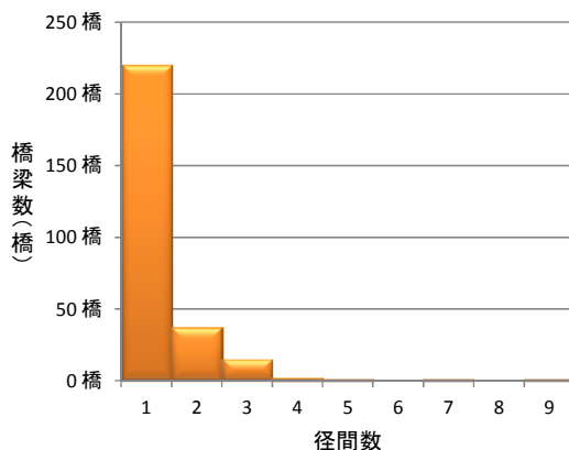
図11 径間数別橋梁数
