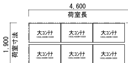
【平面図】
