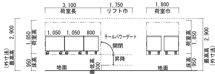
【側面図】
