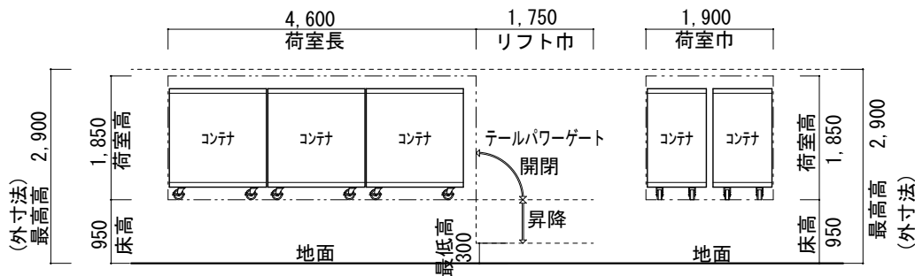
【側面図】
