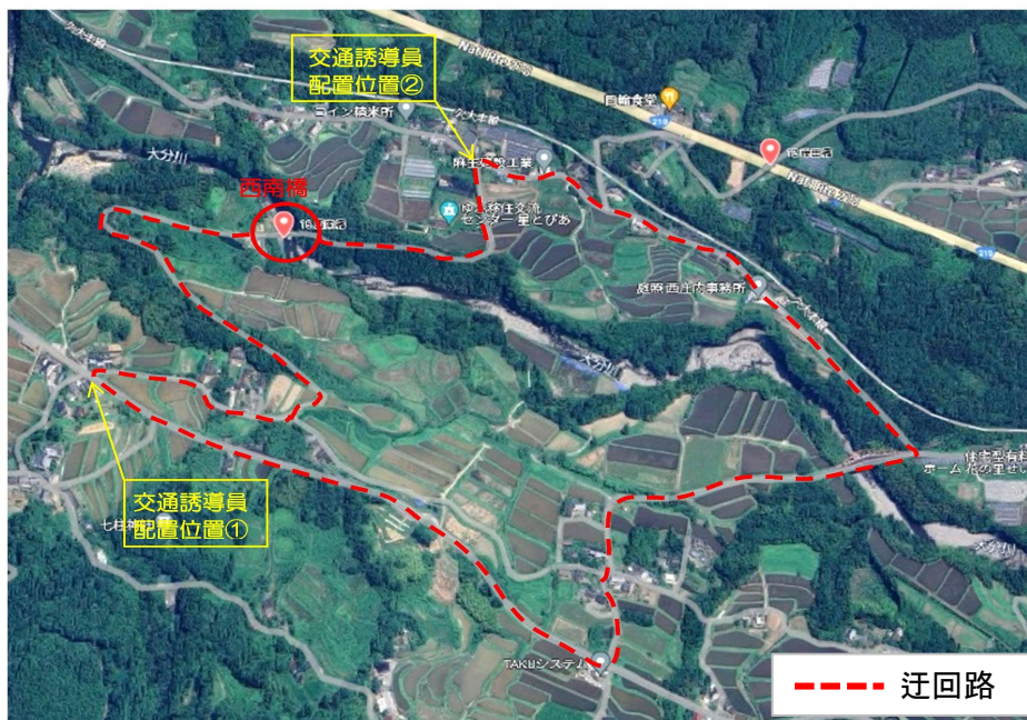
【西南橋 迂回計画図】
