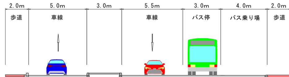
バスのりば横断図
