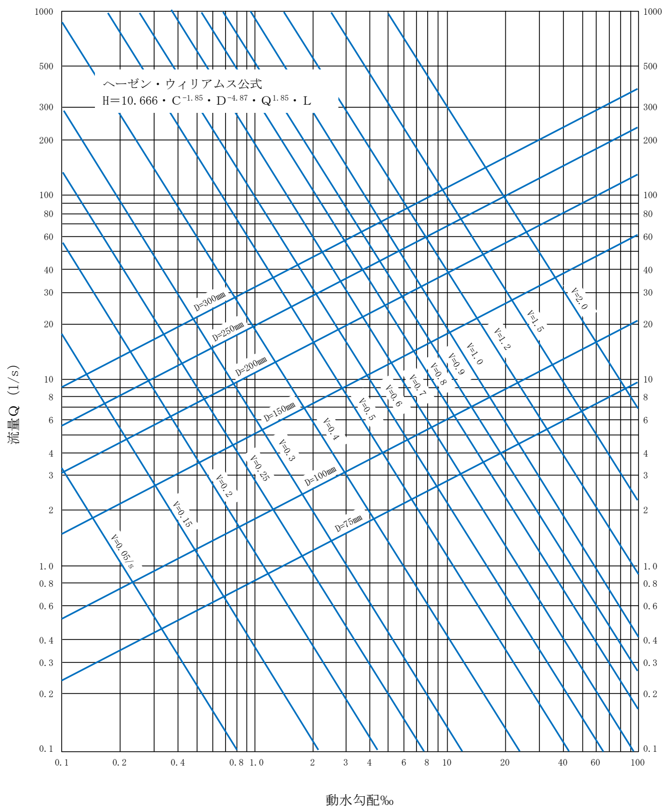
ヘーゼン・ウィリアムス公式図表
