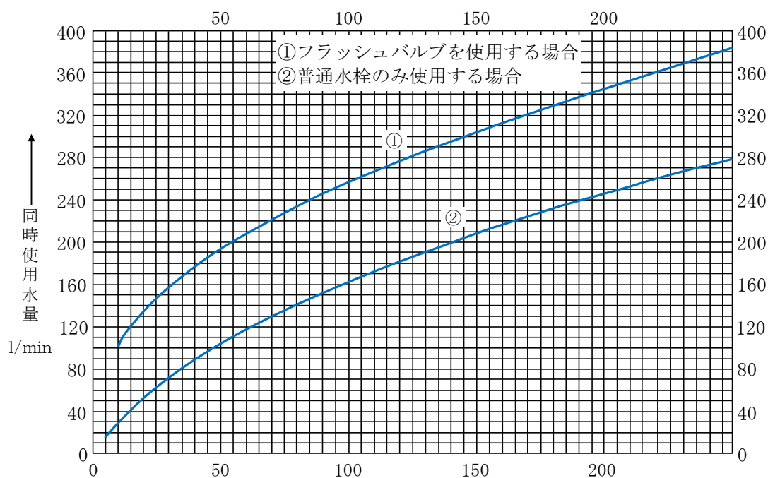
図2－1 給水用具給水負荷単位による同時使用水量図
