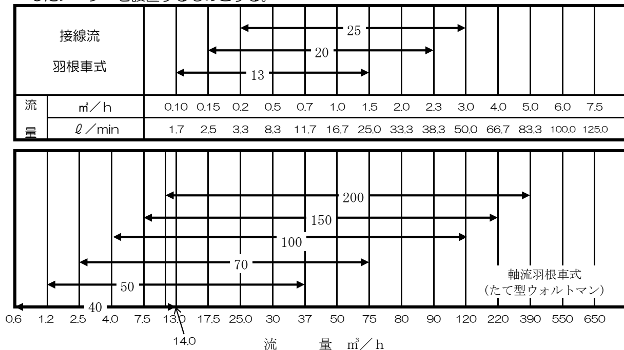
図2-6 時間当たり標準使用範囲表
